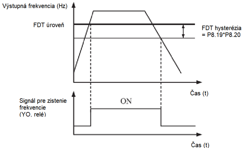
Obrázok 4-14: FDT úrovně
